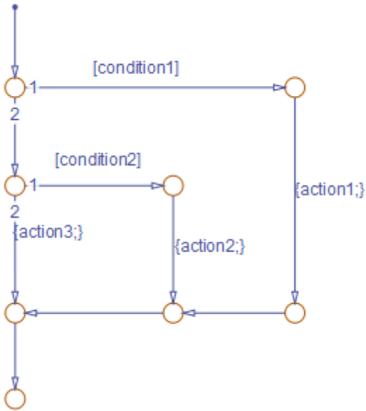
if-elseif-else
